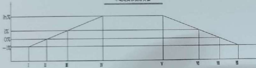
车道超高横坡渐变图
