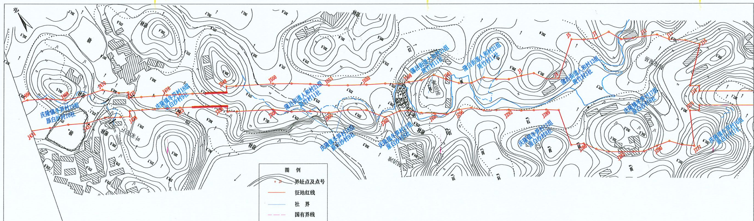
勘测定界图
