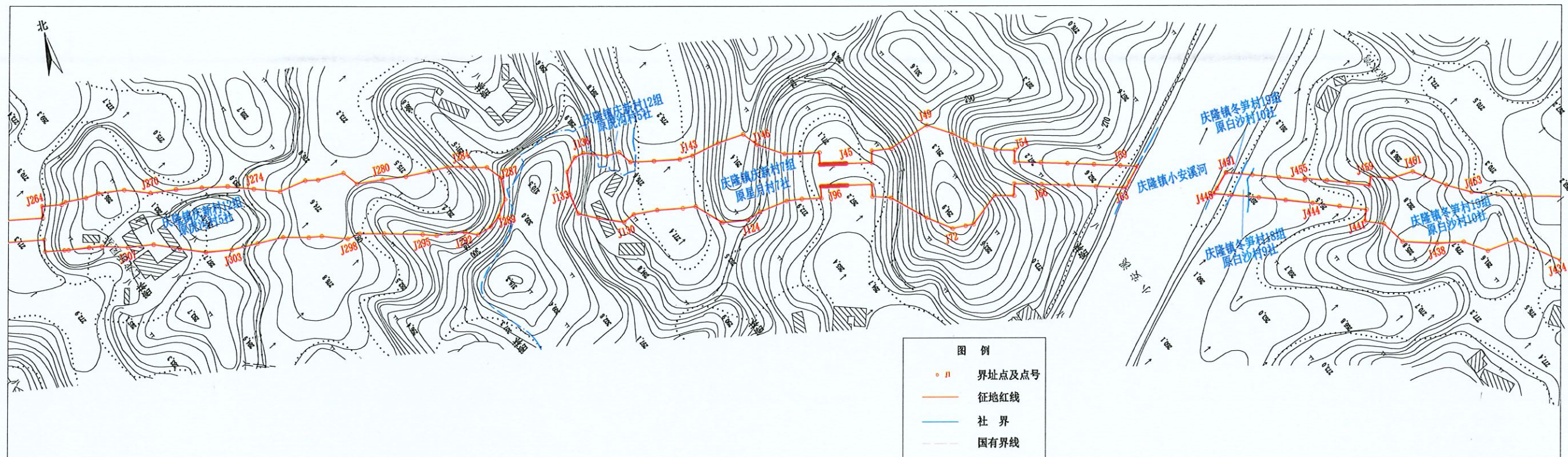
勘测定界图
